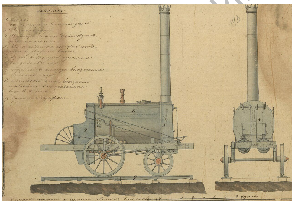
Рис. 6. Чертеж первого паровоза Черепановых. Выполнил Аммос Черепанов
